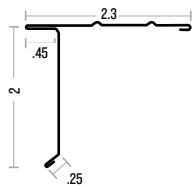
F5S HEMMED DRIP EDGE
