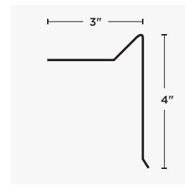
H7 DRIP EDGE
