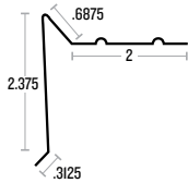
H5 ½ DRIP EDGE
