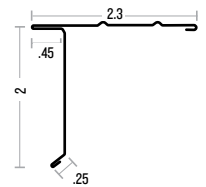
F5S HEMMED DRIP EDGE
